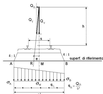
Fig. 5.2.5 - Distribuzione trasversale in rettilineo delle azioni per mezzo delle traverse e del ballast. In figura, Q_h rappresenta la forza centrifuga definita al successivo §5.2.2.3.1
